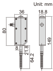
linear gage
